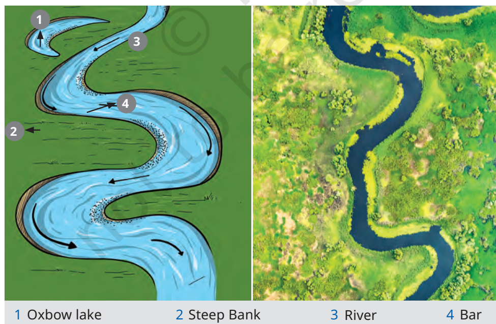
Fig. 2.11. Meander
