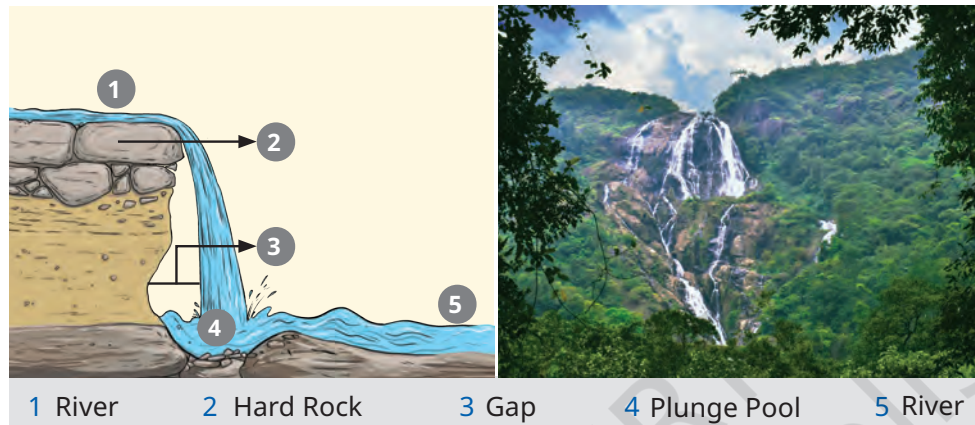
Fig. 2.10. Waterfall
